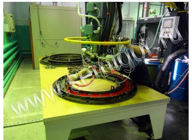
Заполнение формы полиуретаном
